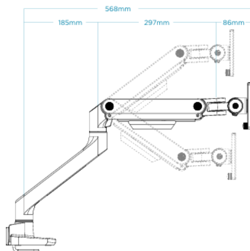
Arm Dimensions
