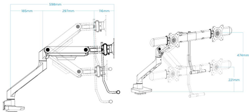
Arm Dimensions
